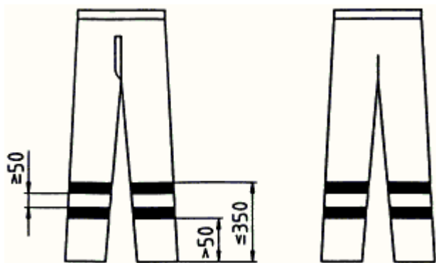
Abb. 11: Ausführungsbeispiele von Warnkleidung der Klasse 1 bis 3
